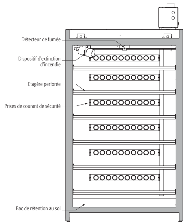
Vue en coupe
