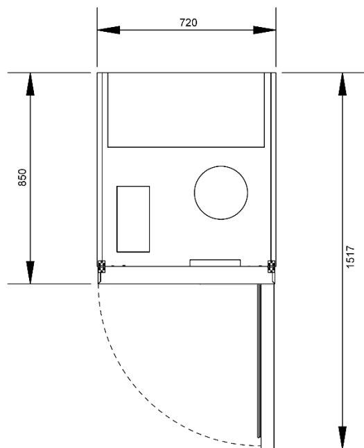
Dessus
