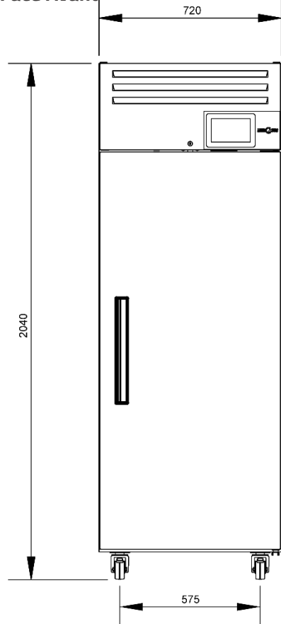
Face Avant
