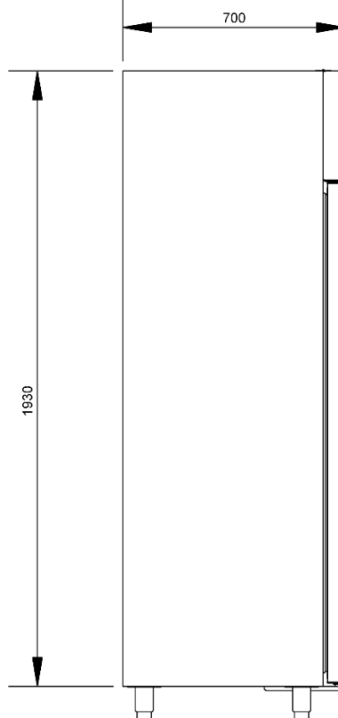
Latérale
