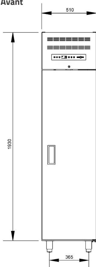
Face Avant
