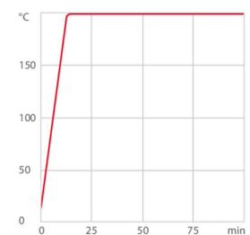
Temps de refroidissement Medium: Etanol
